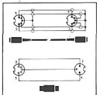
Stereo-Tonleitung K 541 Verbindungskabel Stereo-Radio bzw. Verstärker-Stereo-Tonbandgerät.
