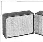
Stereo-Lautsprecherkombination W 82 Die perm. dyn. Oval-Lautsprecher, Durchm. 15,5 x 24 cm, weisen einen Frequenzumfang von 50–15 000 Hz auf und sind mit je 5 Watt belastbar. Anpassung 8 Ohm. Abmessungen: Geschlossen 29 x 40 x 30 cm, Einzelbox 29 x 40 x 15 cm.
